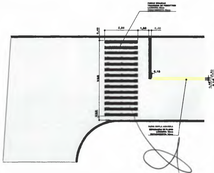
DETALHAMENTO - SINALIZAÇÃO HORIZONTAL SEM ESCALA
