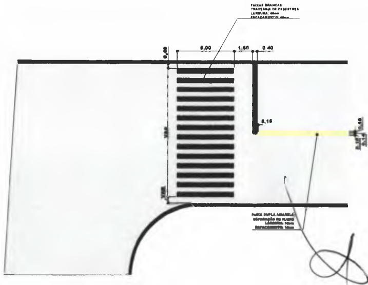
DETALHAMENTO - SINALIZAÇÃO HORIZONTAL SEM ESCALA
